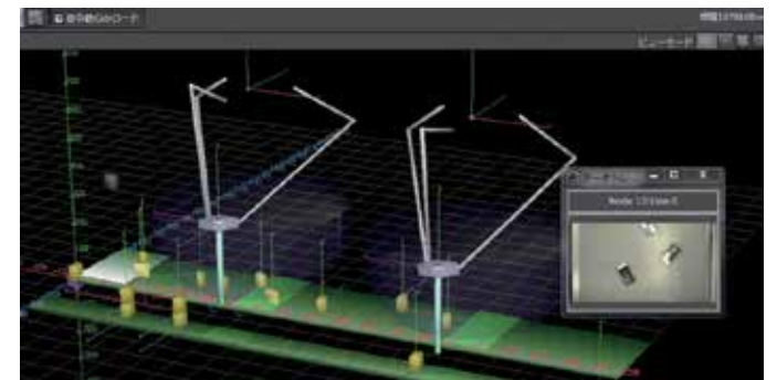
Моделирование системы технического зрения Инспекция и измерения систем технического зрения можно моделировать в Sysmac Studio.
