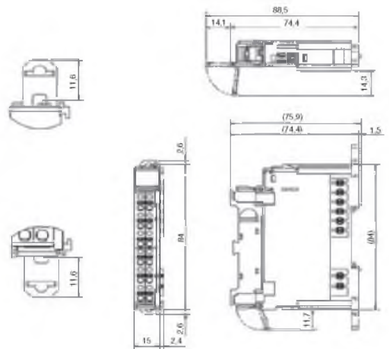
Модули входов/выходов SmartSlice — GRT1_
