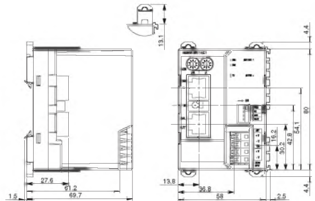
Модули входов/выходов SmartSlice — GRT1_
