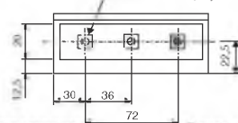
② SGLFW-20A120A□□ — 3 х отв. M4, глубина 5,5
