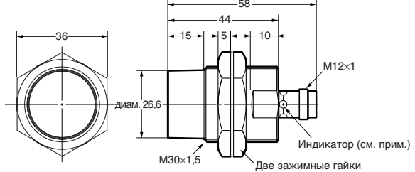
E2A-M30KN20-M1-□□/E2A-S30KN20-M1-□
